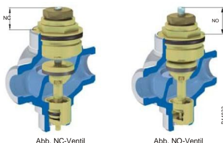
Abb. NC-Ventil
